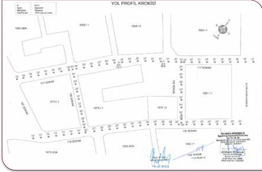
Aktepe Mahallesi 116 ve 117 Sokak Yol Profili (Krokisi)
